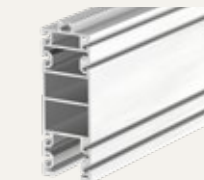
AluvarioPRO Traverse XXL 254 x 89 mm für Teleskopdeck-Rollenkasten
