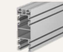
AluvarioPRO Traverse XXL Pro 239 x 89 mm für Pools mit Beckenrandhöhe bis 150 mm
