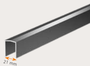
UniAbdeckleiste für 45° Elemente oder andere Füllungen, Aufnahme 21 mm
