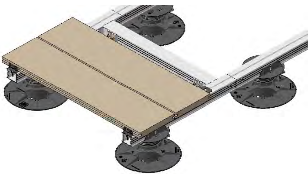
Dielen auf Alusystem und Stelzlager
